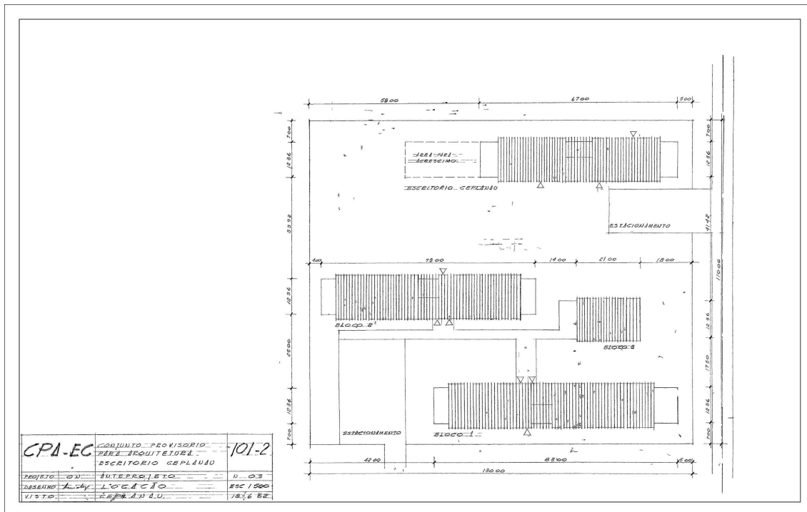
Figura 2: Anteprojeto – Locação. O “Escritório do Ceplan” está na parte de cima do desenho (1962).
