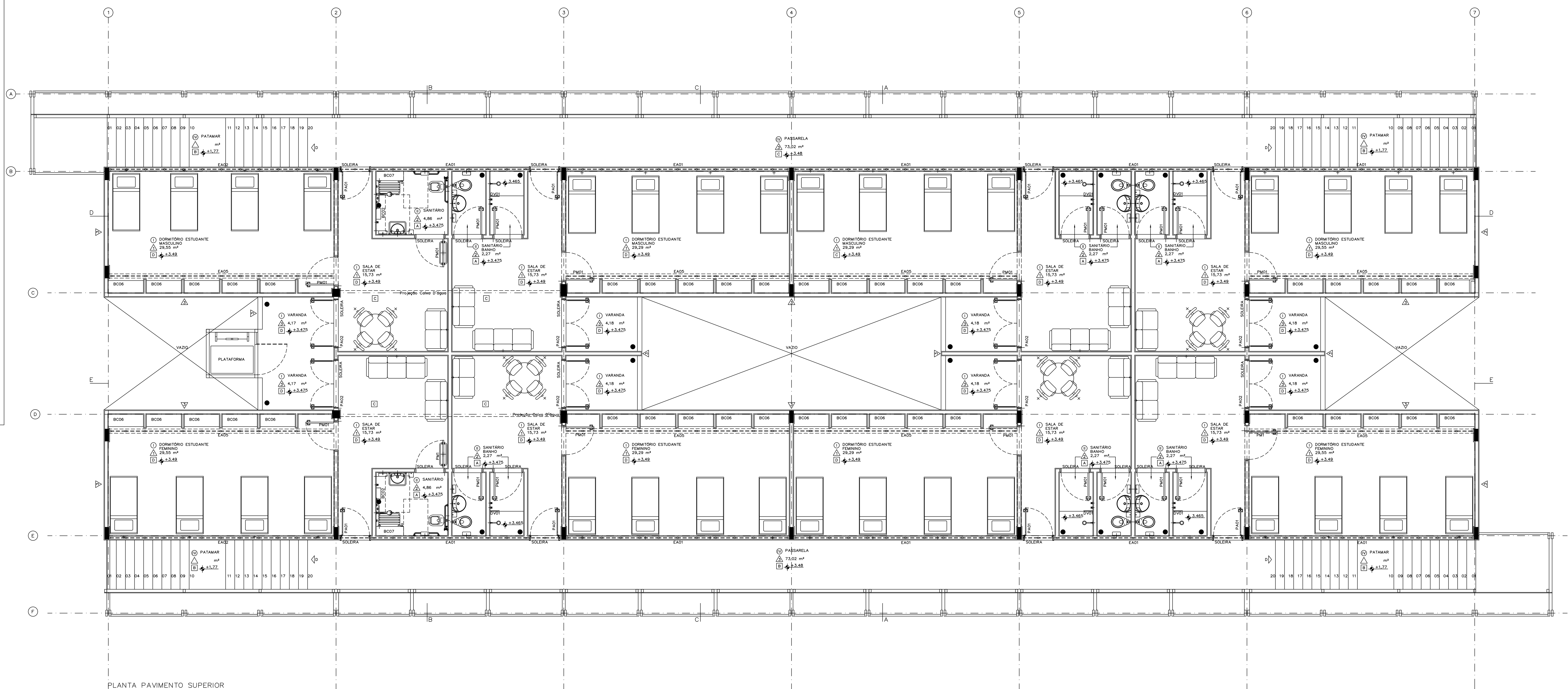
PLANTA PAVIMENTO SUPERIOR ESQ.: 1:50 ÁREA: 612,06 m²
