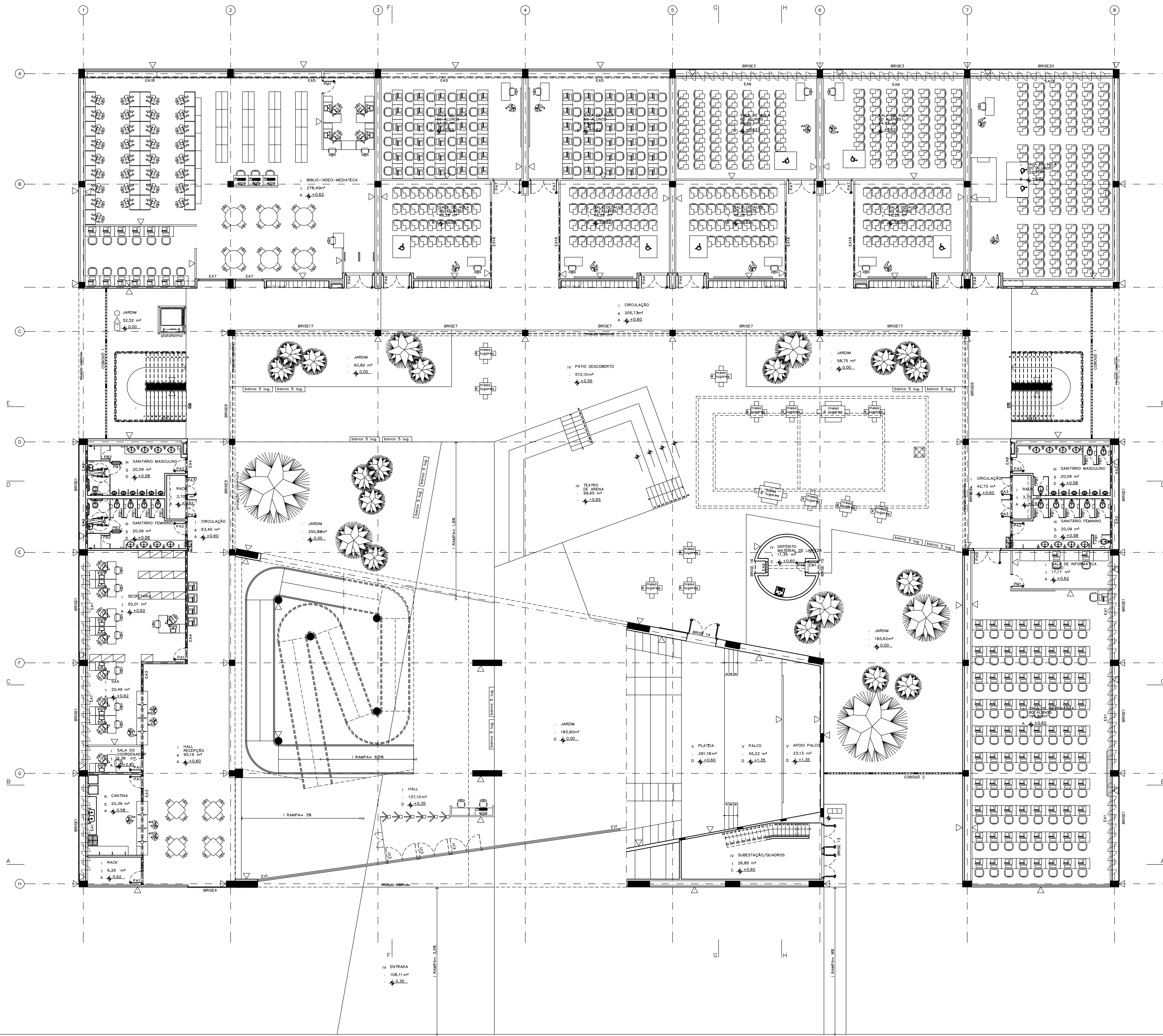
PLANTA PAVIMENTO TÉRREO ESCL: 1:100
