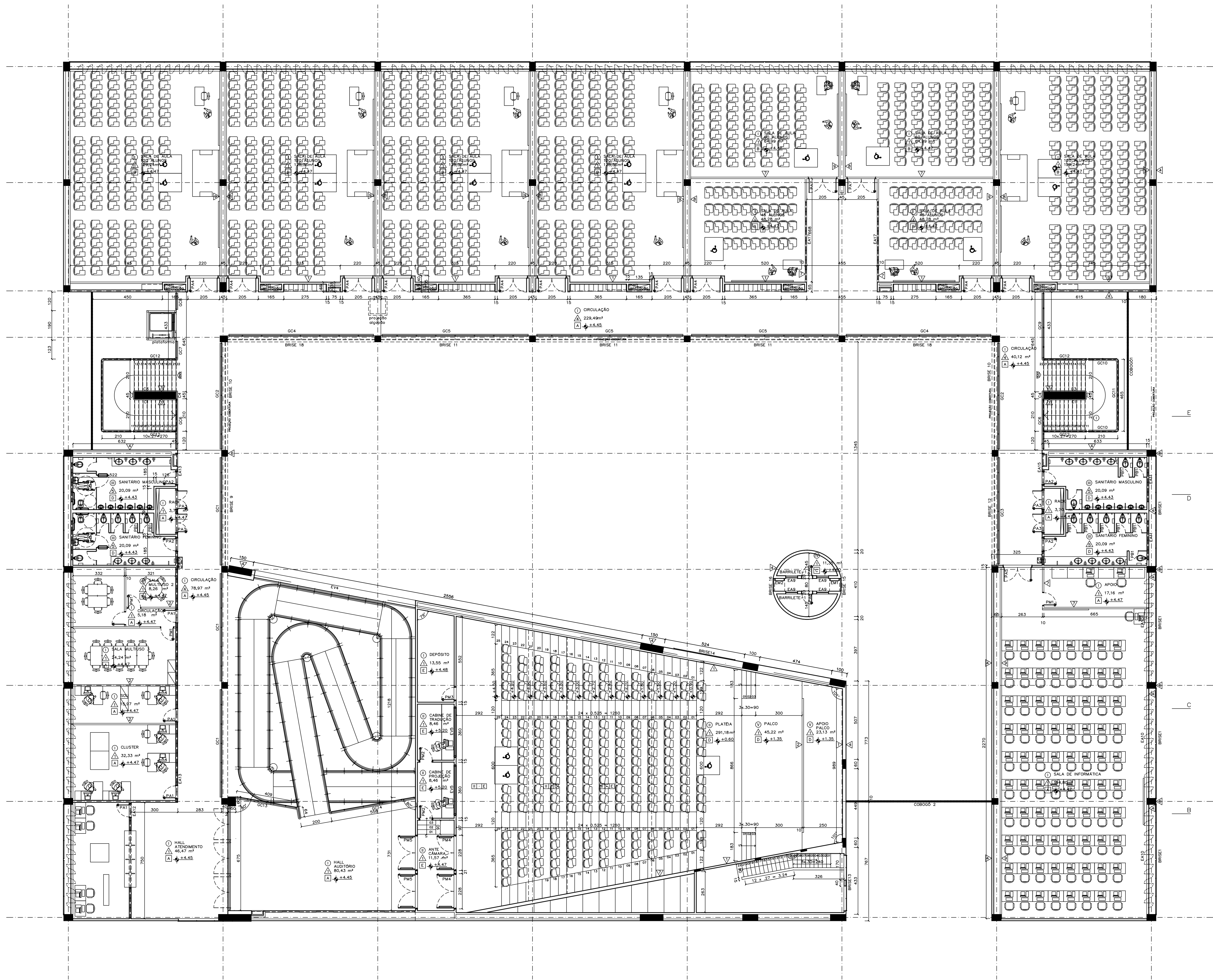
PLANTA PAVIMENTO SUPERIOR
